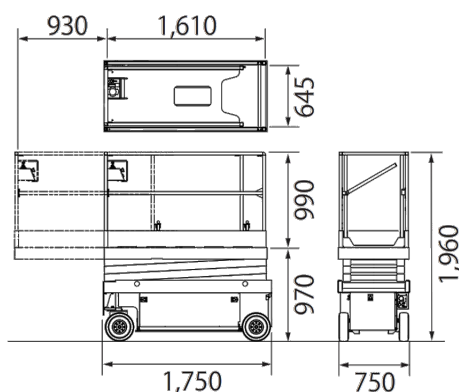
■ENTL061-2 本体寸法図
